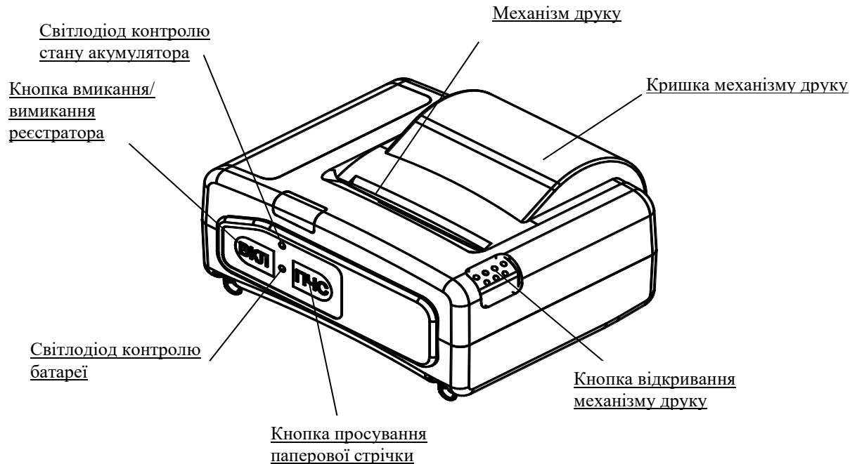
Рисунок 1 – Зовнішній вигляд реєстратора
